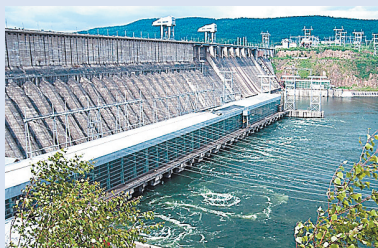
БРАТСКАЯ Установленная мощность: 4500 МВт Высота плотины: 125 м Где находится: р. Ангара, Иркутская область
