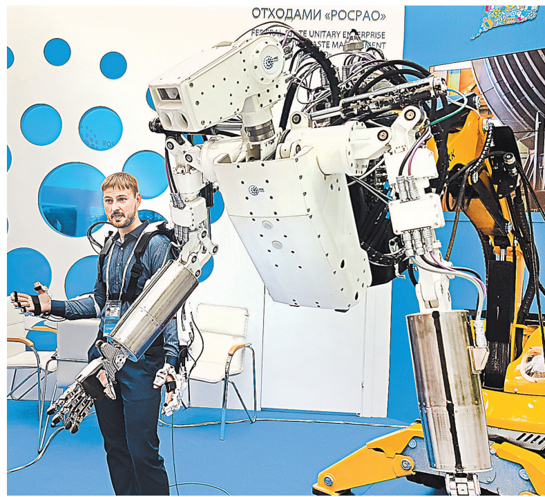
Такие роботы сегодня работают с радиоактивными отходами.
